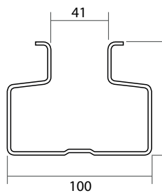
Bastidores en fondo 700 y 850, consultar Uprights with 700 and 850 depth, please consult / Echelles de fond 700 et 850, consulter
