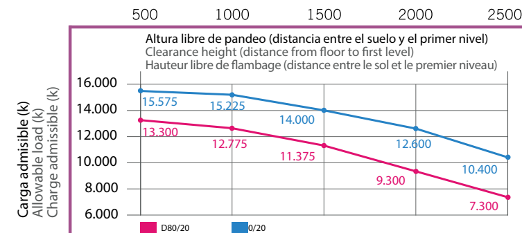
Bastidores en fondo 700 y 850, consultar Uprights with 700 and 850 depth, please consult / Echelles de fond 700 et 850, consulter
